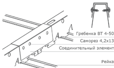
Узел установки соединительного элемента гребёнки
