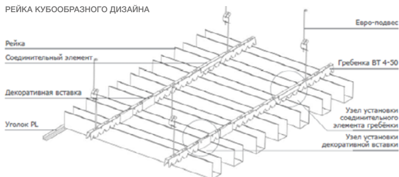
РЕЙКА КУБООБРАЗНОГО ДИЗАЙНА
