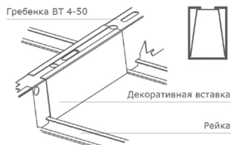
Узел установки декоративной вставки
